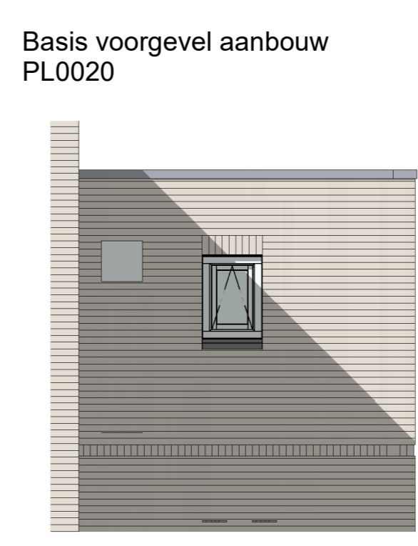
VG5031 - Badkamerraam in voorgevel aanbouw
