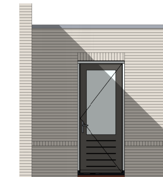
VG5026 - Enkele loopdeur in voorgevel gespouwd berging/aanbouw
